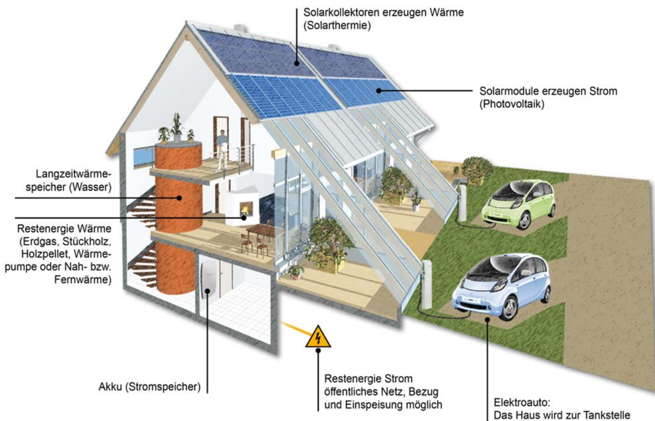
Abb. 1: Prinzipdarstellung eines energieautarken Einfamilienhauses.
